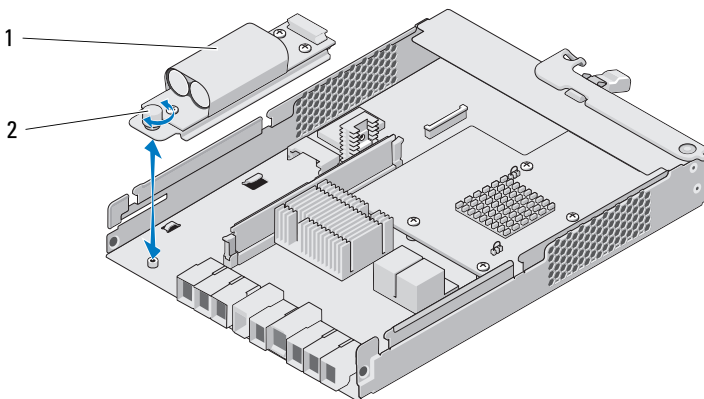
图 16-10. 卸下和安装 RAID 控制器模块备用电池装置
